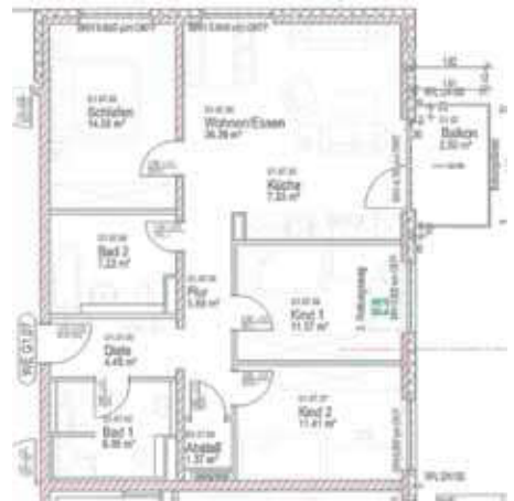
Grundriss WE Nr. 29 (in der Bauakte als G1.07 bezeichnet)
