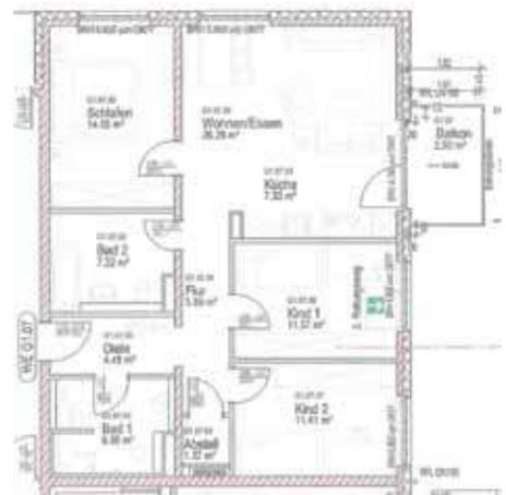
Grundriss WE Nr. 29 (in der Bauakte als G1.07 bezeichnet)
