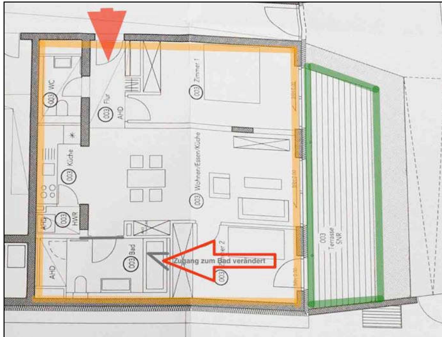
Grundriss Wohnung 003
