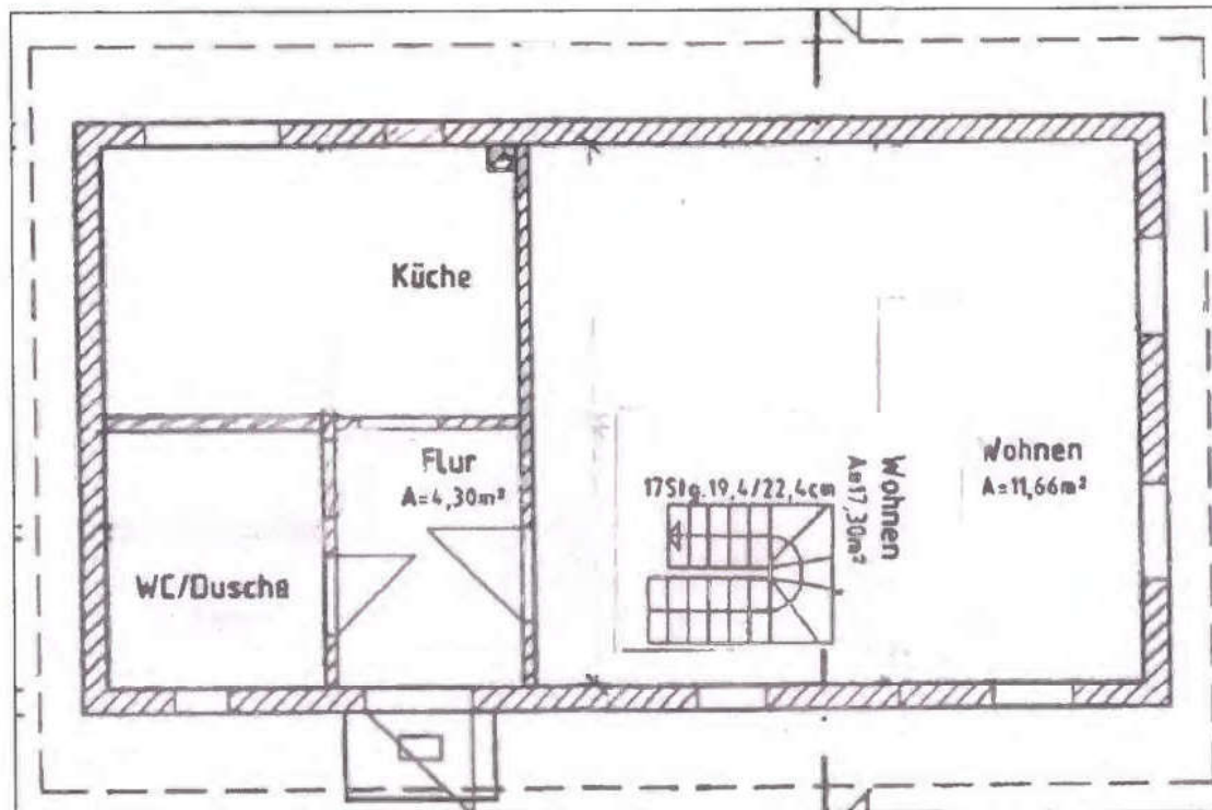
Grundriss ohne Wintergarten nach den Gegebenheiten bei der Ortsbesichtigung. (eigene Darstellung, ohne Maßstab)
